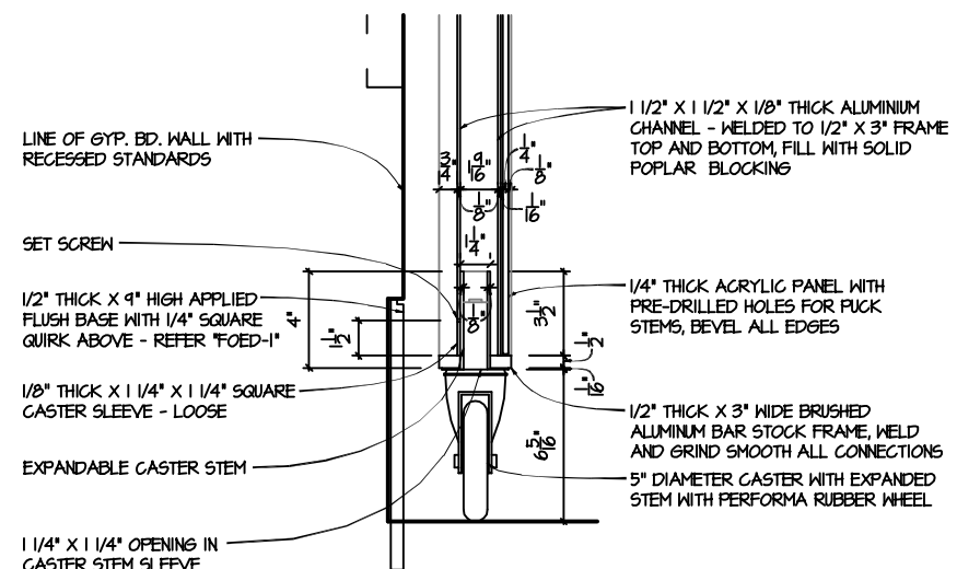
A-3 DETAIL SCALE: 3/4"=1'-0"
