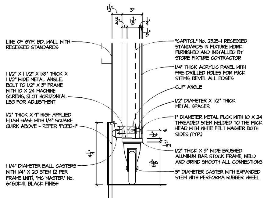
A-2 DETAIL SCALE: 3/4"=1'-0"
