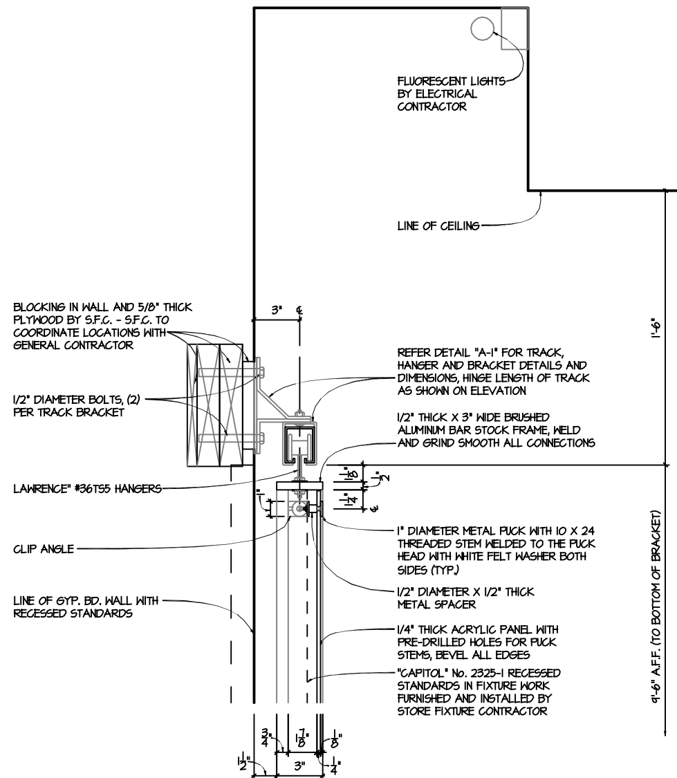
A-1 DETAIL SCALE: 3/4"=1'-0"
